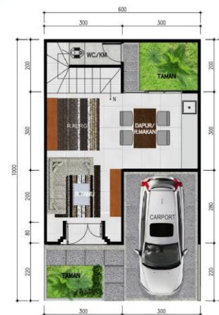
DENAH LT.1
